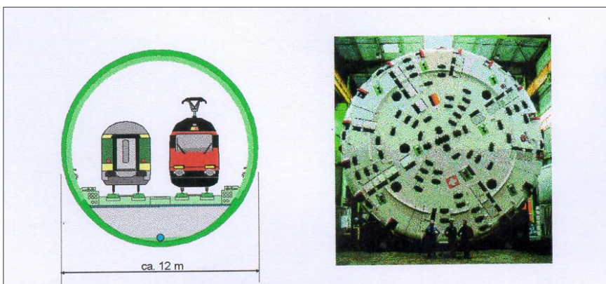
Normalprofil und Tunnelbohrmaschine
