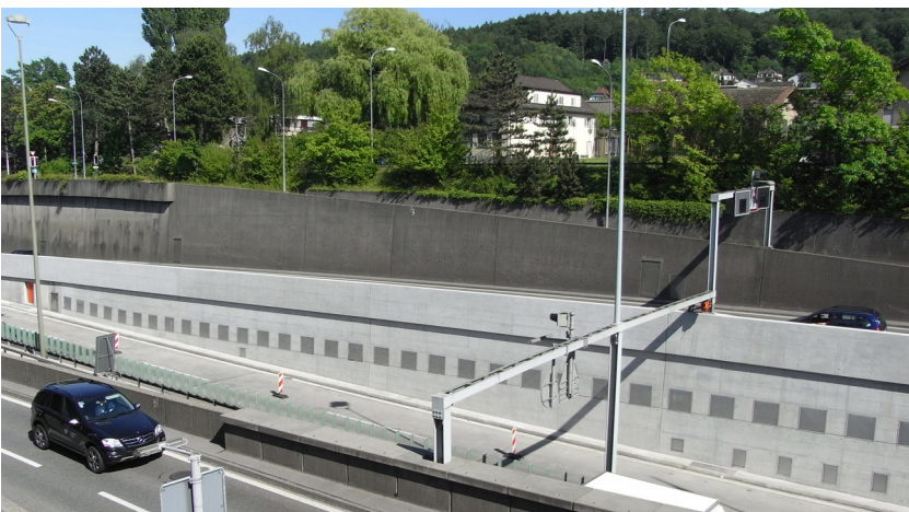
Pfahlwand nach der Instandsetzung
